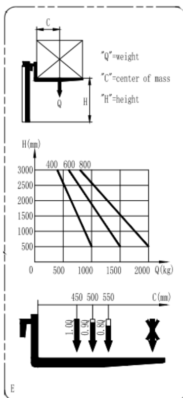
Рис. 2 – Кривая грузоподъемности
